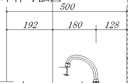
手洗い器本体寸法図
