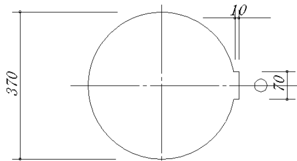
カウンター開口寸法図
